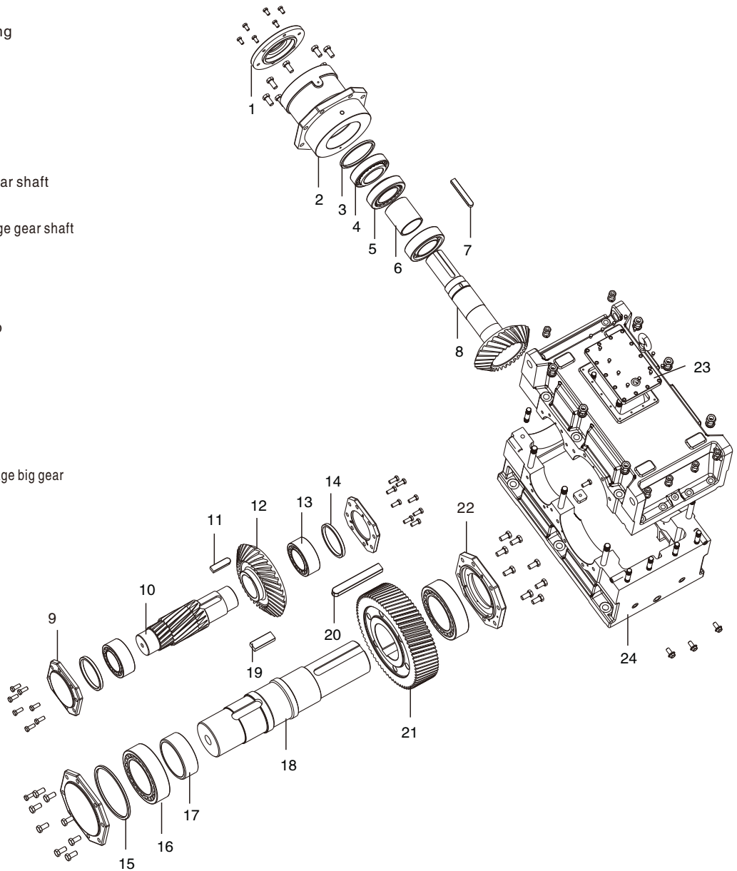
AB系列结构图:/AB series structrue drawing:
